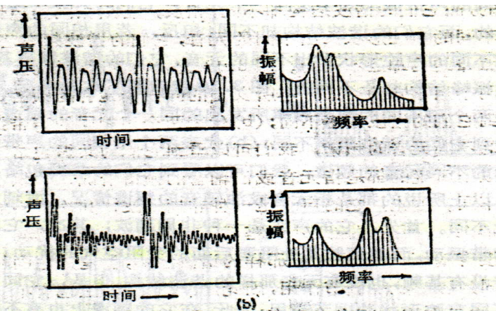
*图 3.10 (a) 用不同的声带频率所发的同一元音的波形和频谱 (b) 用相同的声带频率所发的不同元音的波形和频谱
